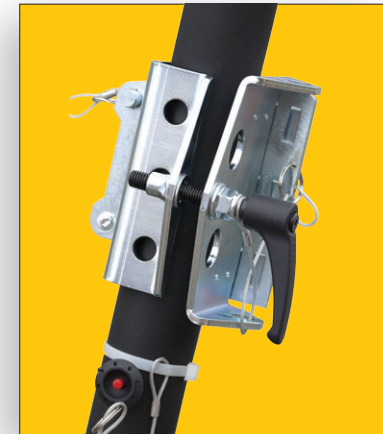
Tripod TM 15 & TM 15 MINI & TM16 ROUND PROFILE Ø60 mm
